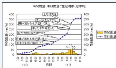
H14釜石市土石流での雨量と前兆現象 作成：井良沢道也
